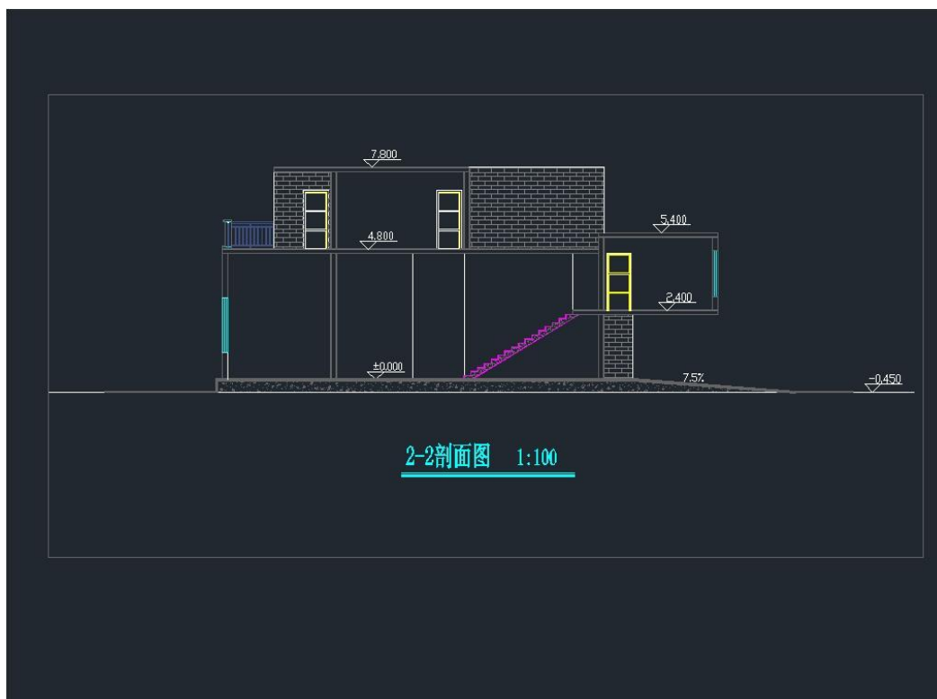
别墅后视图
