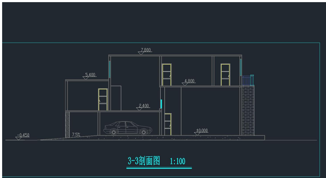
别墅左视图
