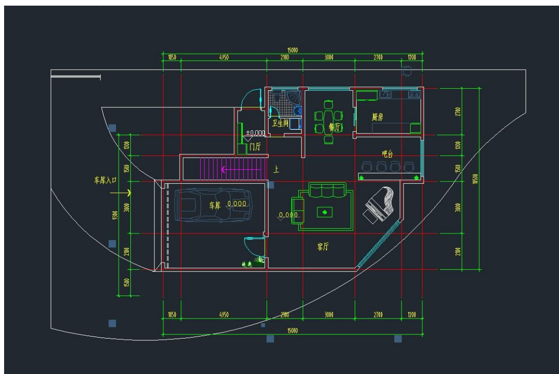
別墅一层户型图
