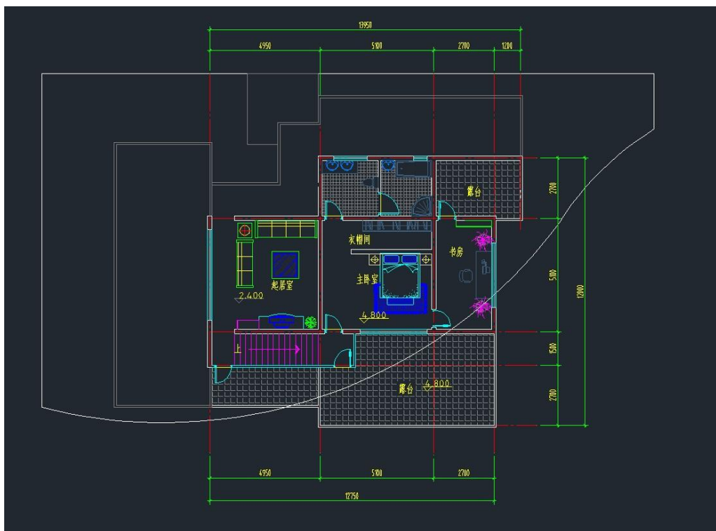
别墅三层户型图
